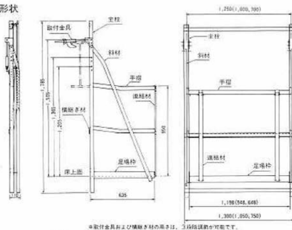
取付金具の規格(鉄製) (単位: mm)
