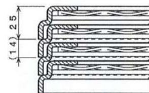
[フレーム断面図]
